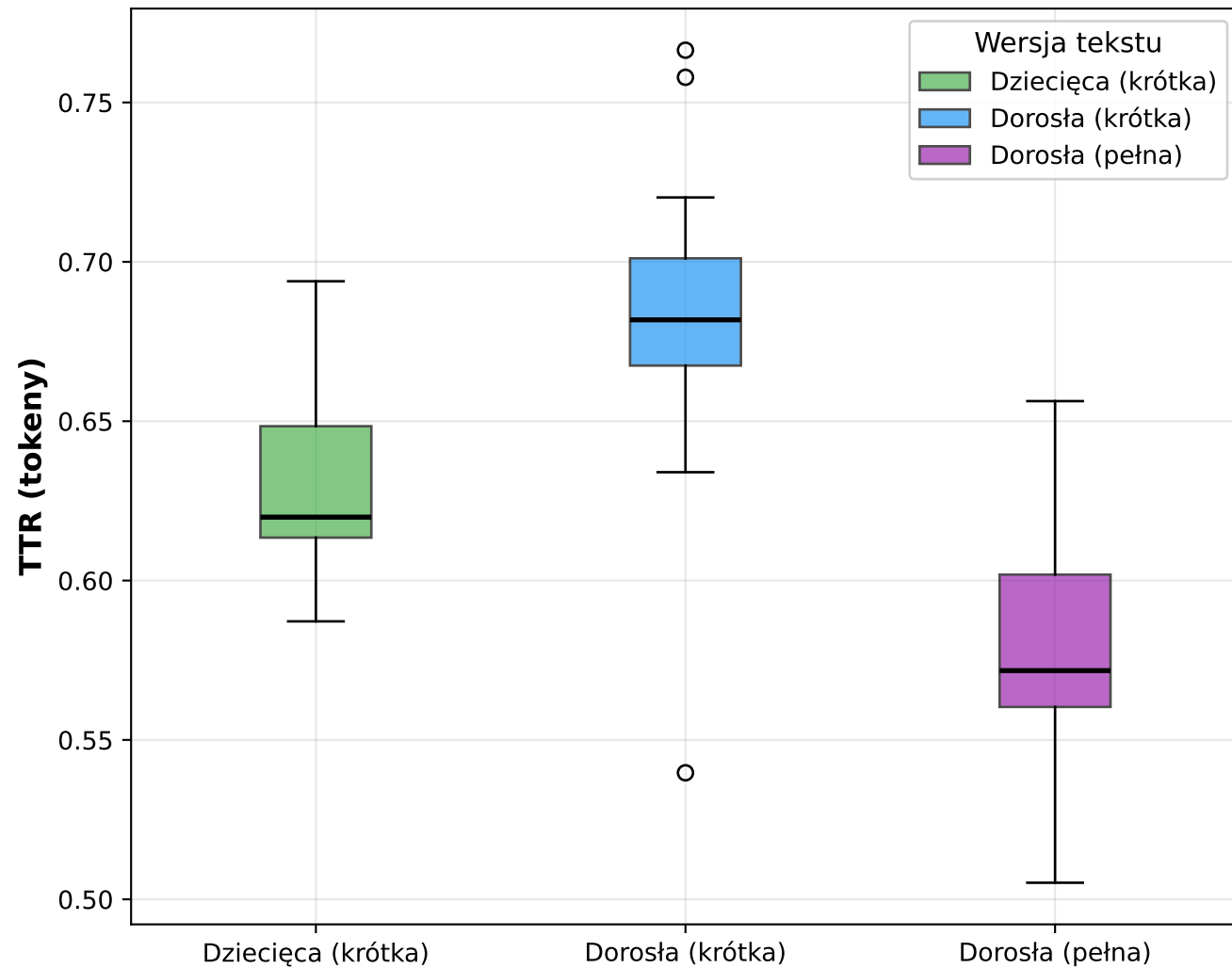
Rozkład TTR dla tokenów (boxplot)
