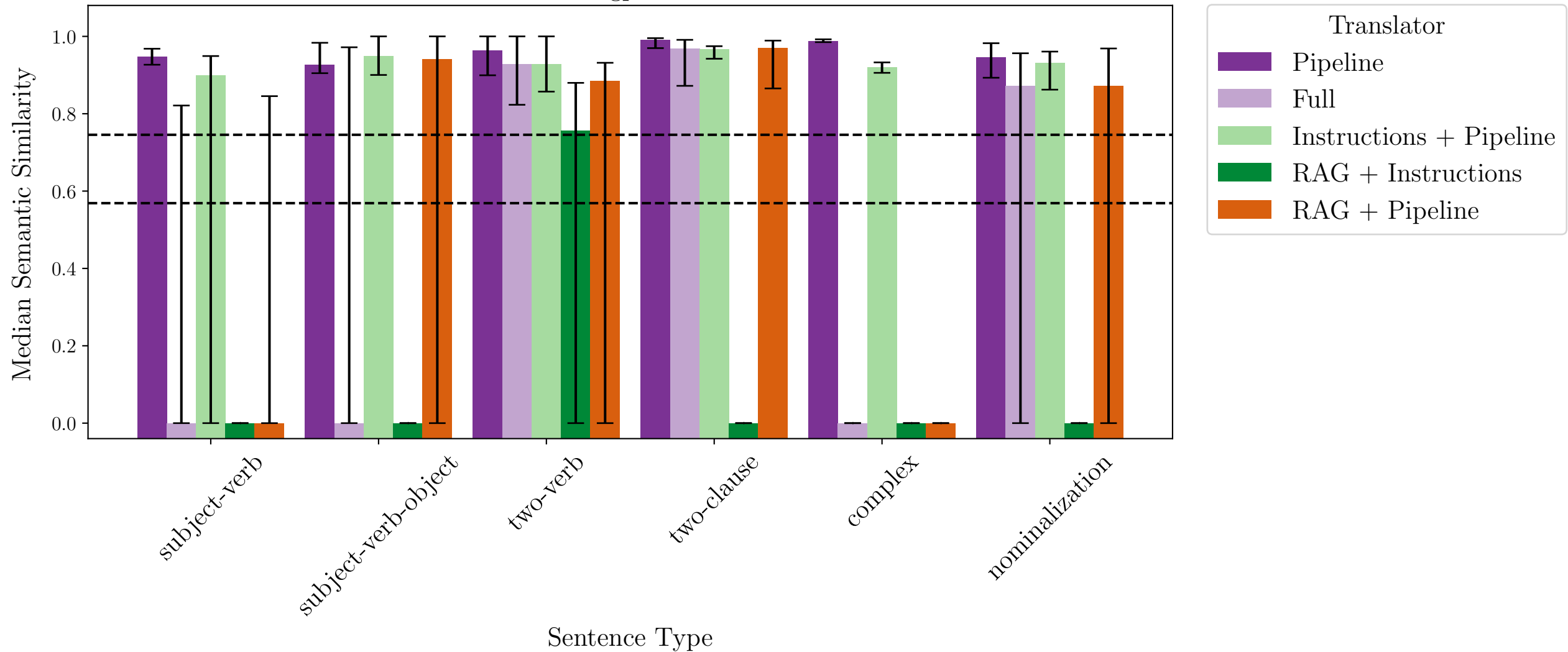
Model: gpt-4o-mini
