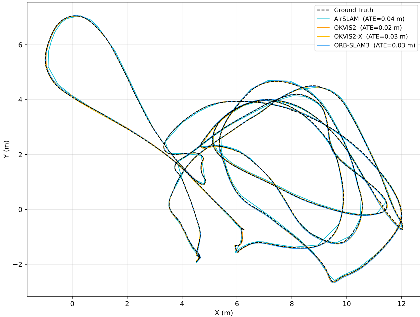
Trajectory comparison — euroc_mav / MH_03_medium
