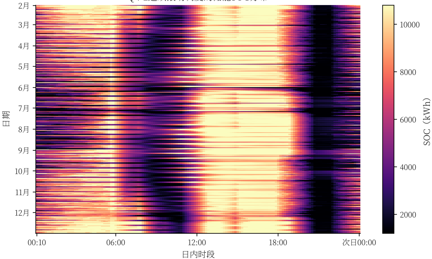
Q4-2连续滚动调度的储能SOC分布
