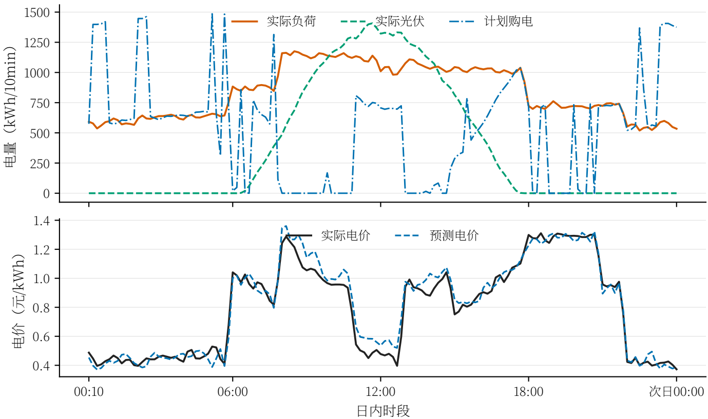
代表日供需与动态电价 (2025-02-25)
