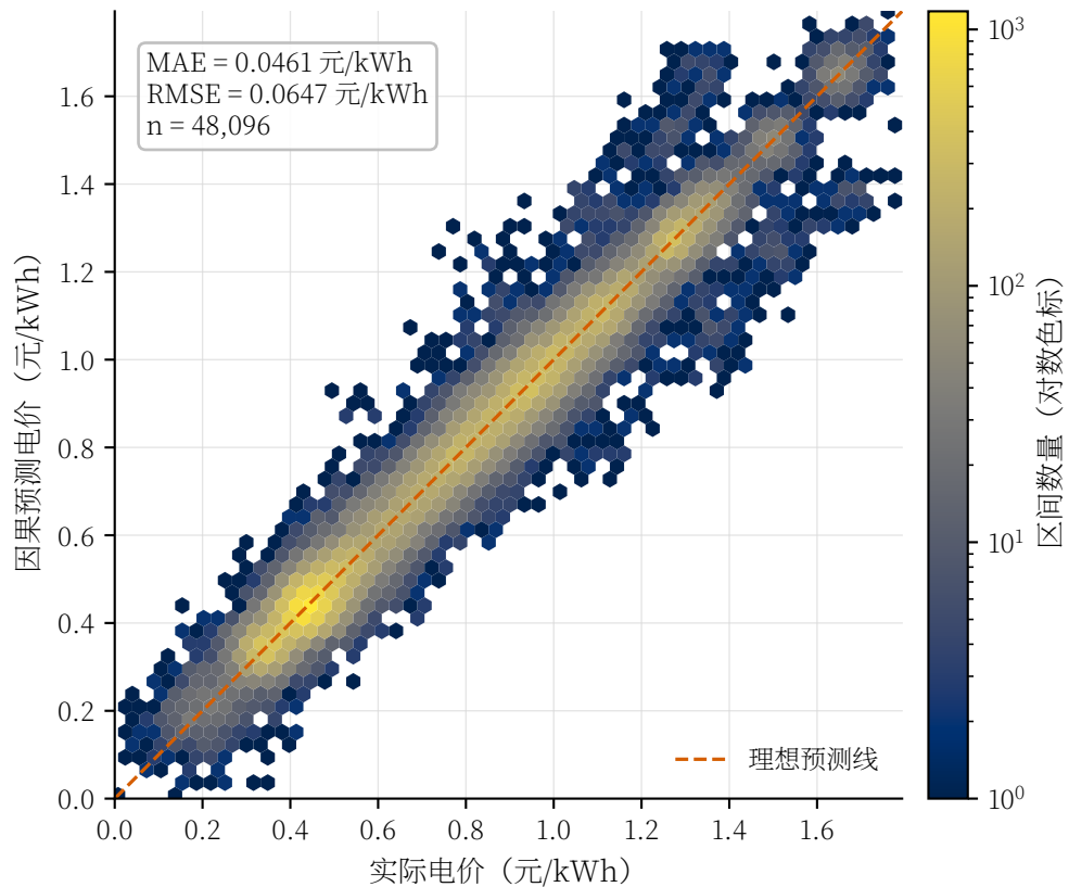
M3执行时点的预测电价与实际电价
