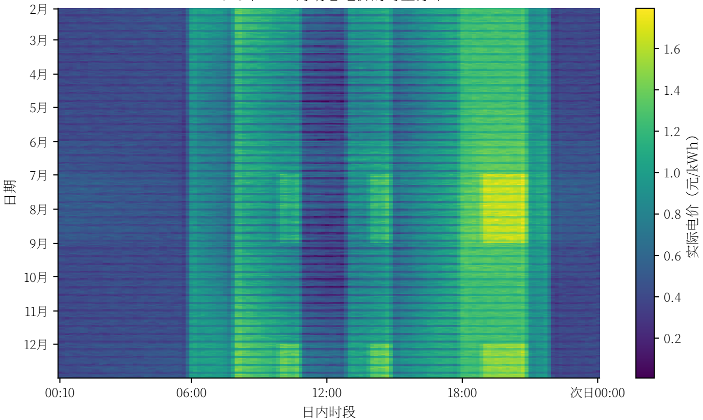
2025年2—12月动态电价的时空分布
