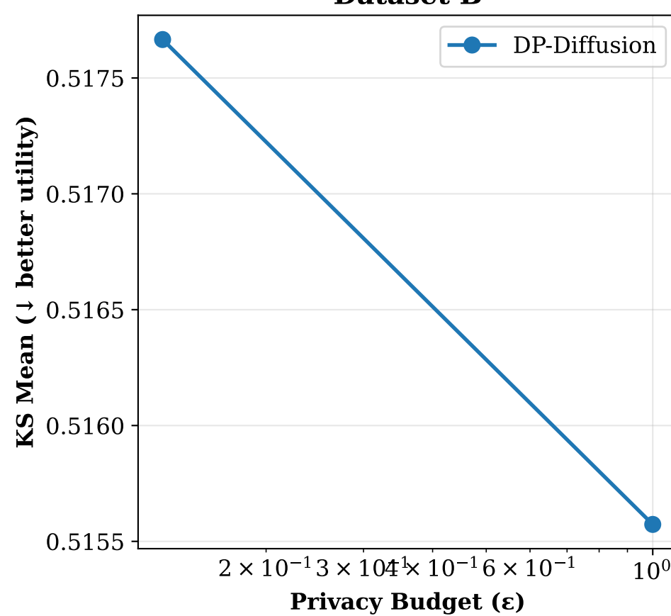
Dataset B
