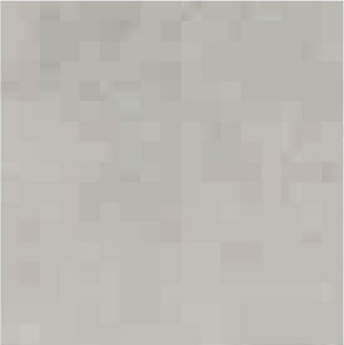
Arenisca Marengo
