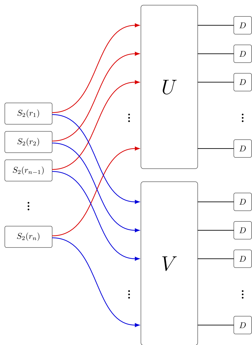
(b) Bipartite GBS
