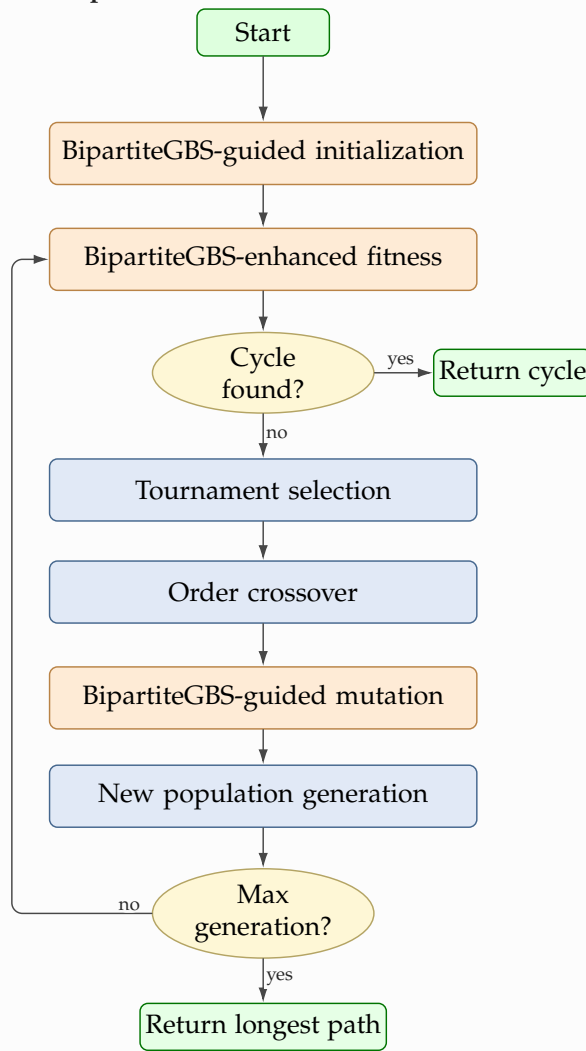
(b) BipartiteGBS-GA
