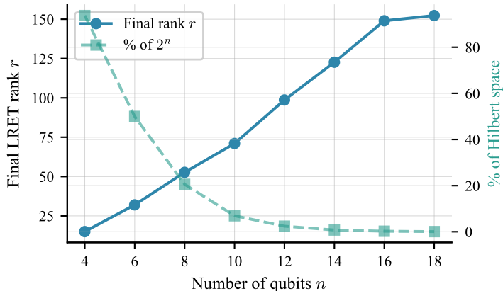
(d) Rank Compression
