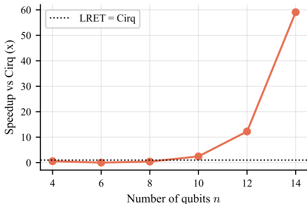
(d) Rank Compression
