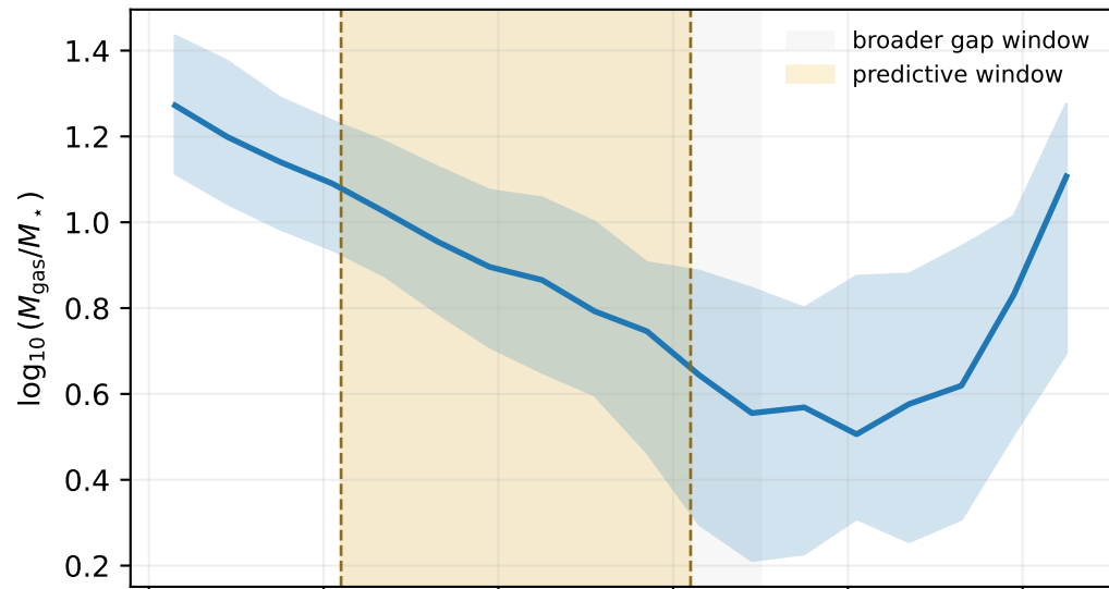
CAMELS-TNG CV
