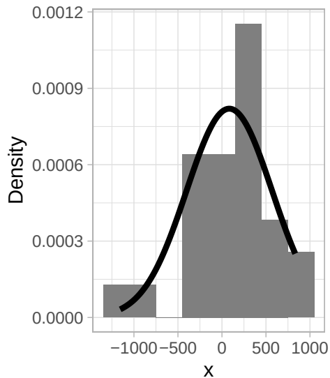
Random normal values
