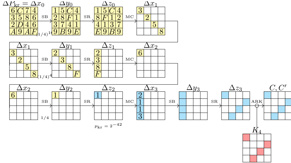
图 4: 扩展视角: 多轮差分 trail 在 SmallScaleAES 中的传播。每轮的活跃 nibble 模式展示了差分如何在 SubBytes→ShiftRows→MixColumns→AddRoundKey 的循环中扩散。
