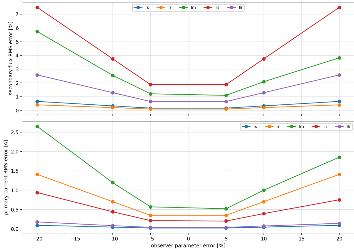
Parameter error sensitivity at 5000 r/min, -220 Nm
