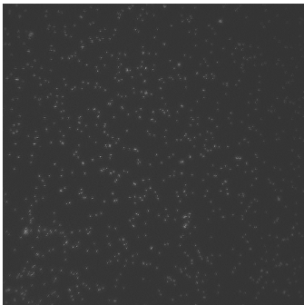
\hat{\mathcal{S}}_{\text{model}}
