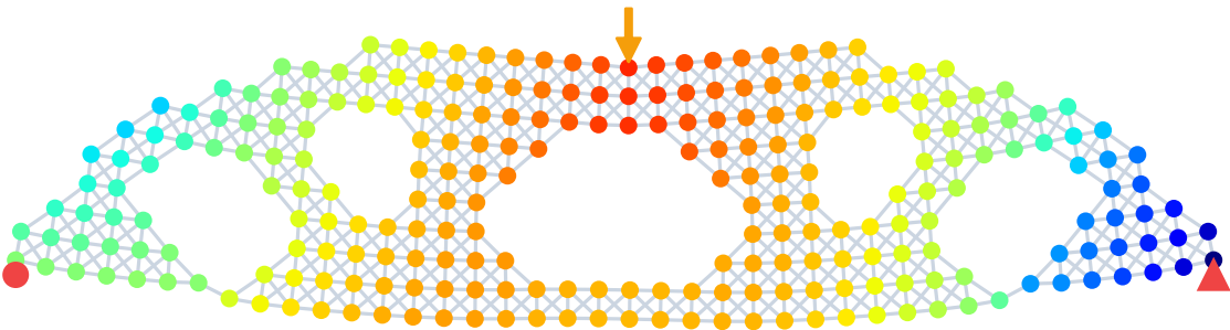
3. Verformung
