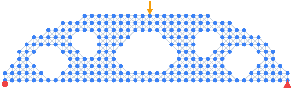
2. Optimierte Topologie
