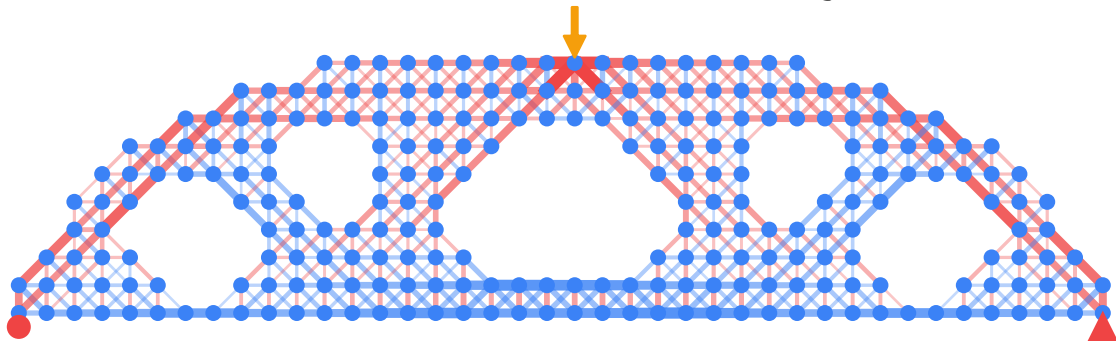
4. Kraftfluss (Rot=Druck, Blau=Zug)
