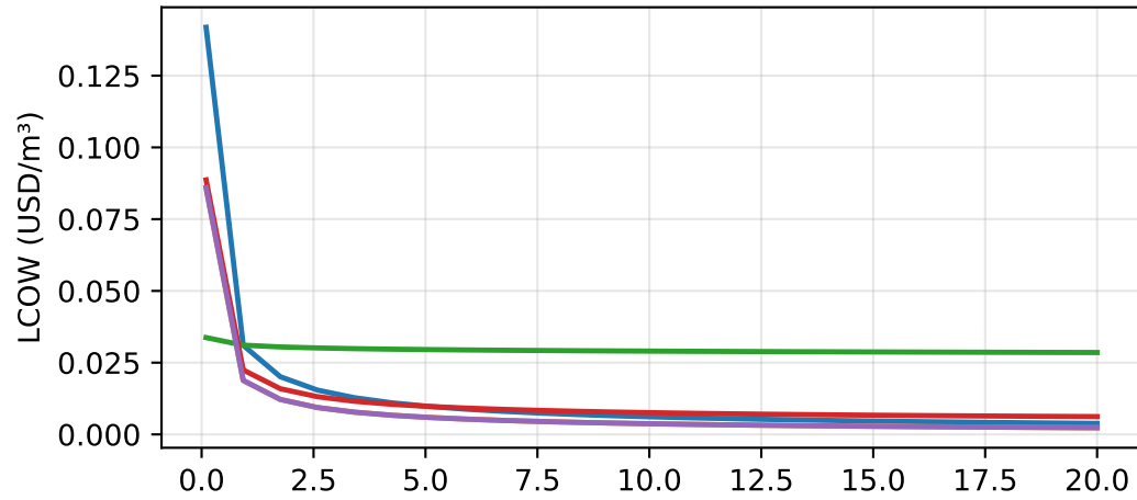
Linear Scale
