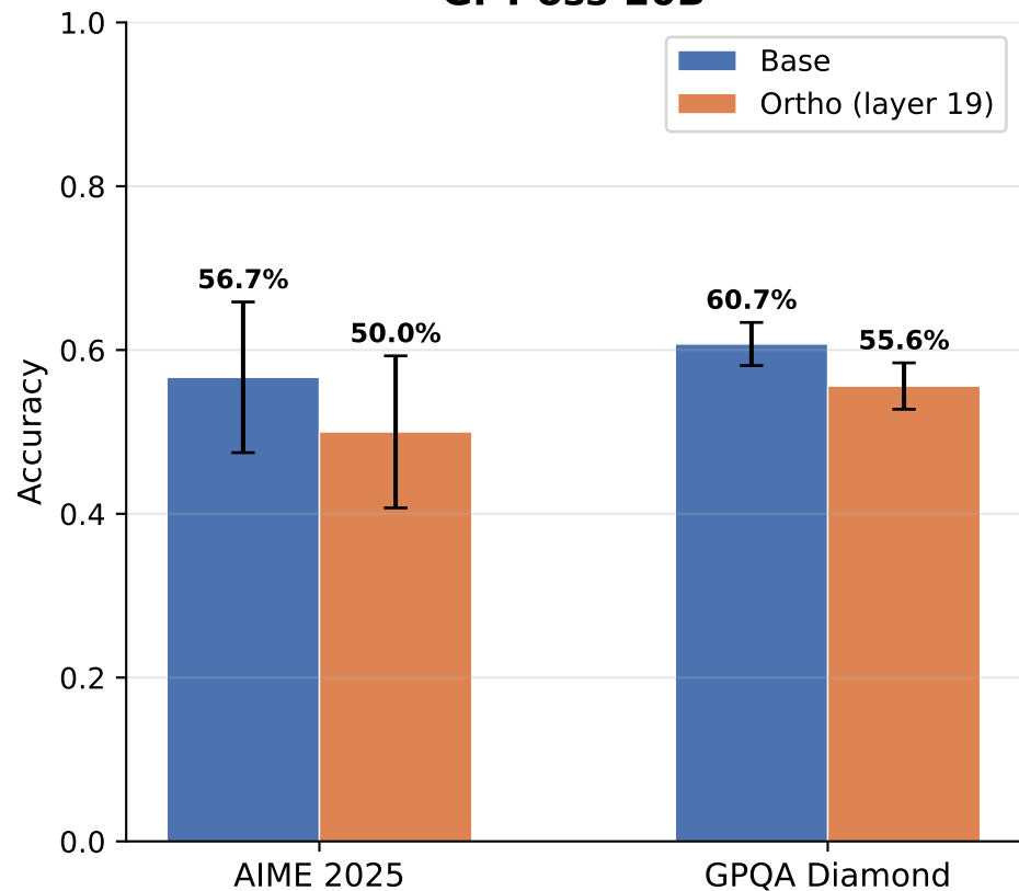
GPT-oss-20B
