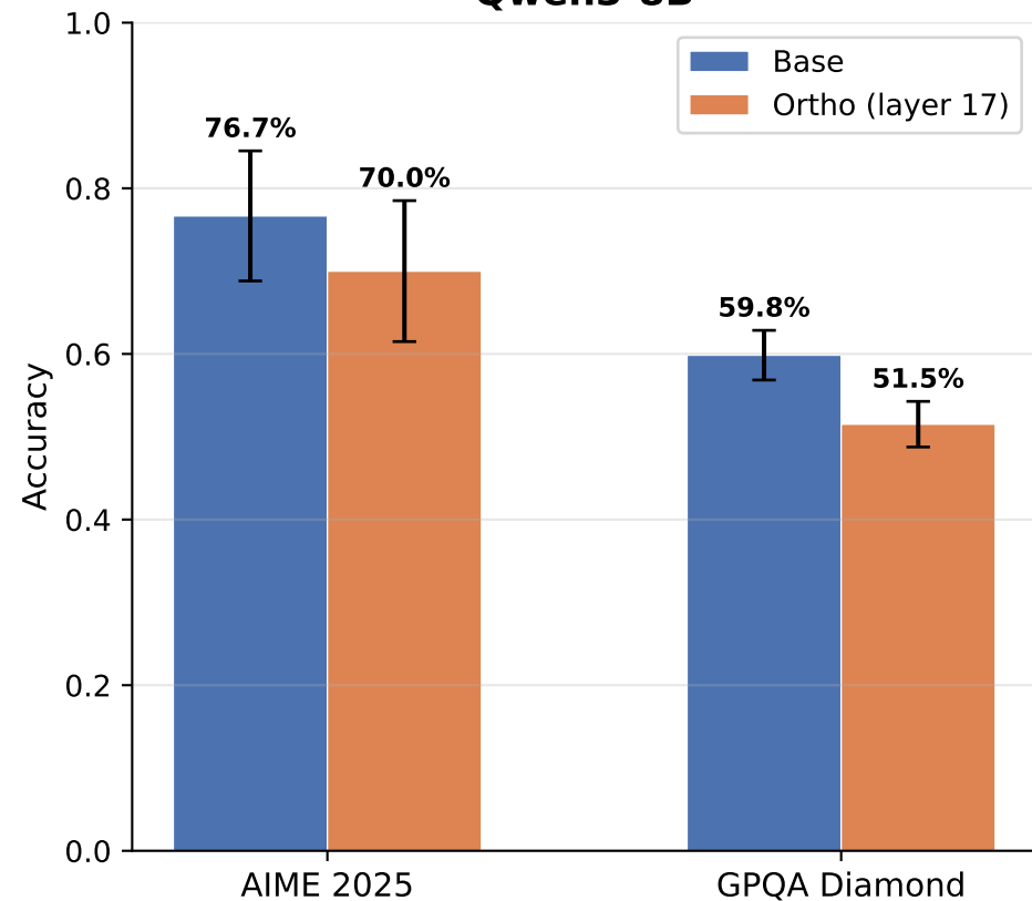
Qwen3-8B
