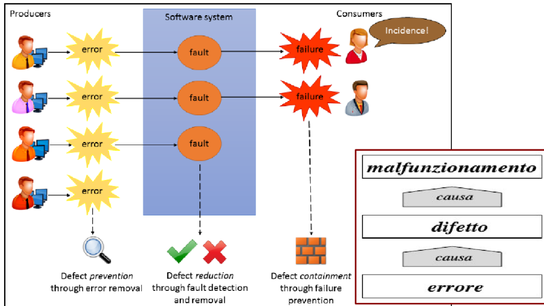
Figura 17.2: Relazione tra error , fault e failure : l'errore umano introduce un difetto nel sistema software, che può manifestarsi all'utente come malfunzionamento osservabile. La figura evidenzia anche tre strategie di intervento: prevenzione degli errori, rilevazione e rimozione dei fault, e contenimento delle failure.
