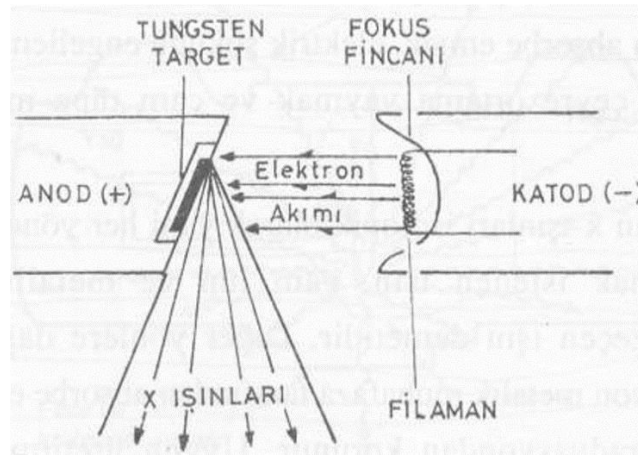
Şekil 26: Sabit Anot Yapısı (58)
