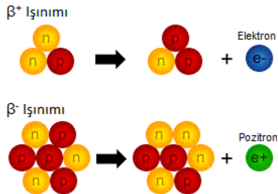
Şekil 11: \beta^- ve \beta^+ Işıını (124)
