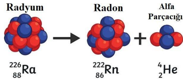
Şekil 8: Radyum elementinin alfa ışıması ile Radon elementine dönüşmesi (17) .
