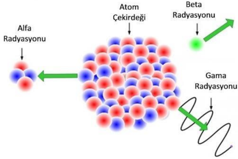
Şekil 1: Alfa, Beta, Gama ışıınları (6) .
