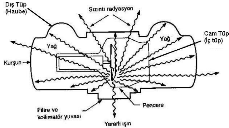
Şekil 19: X-Ray Tüp Yapısı (58)
