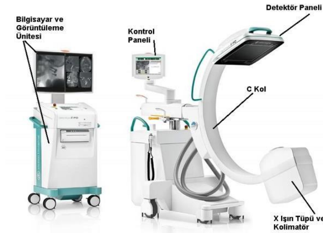
Şekil 35: C Kollu Skopi Cihazı (41)
