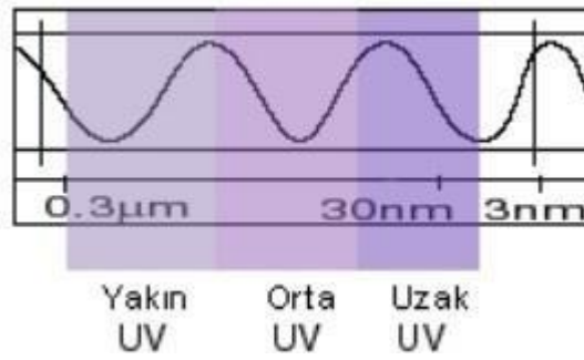
Şekil 12: Dalga boylarına göre yakın, orta, uzak ultraviyole ışını (3) .
