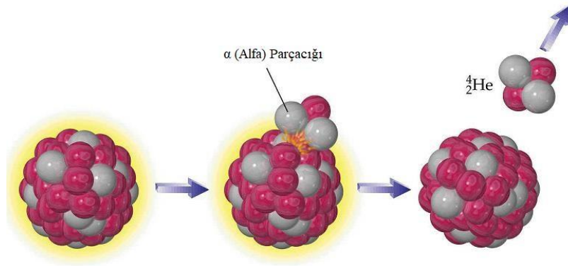
Şekil 6: \alpha (Alfa) parçacığı yada \text{He}^{2+} oluşumu (5) .
