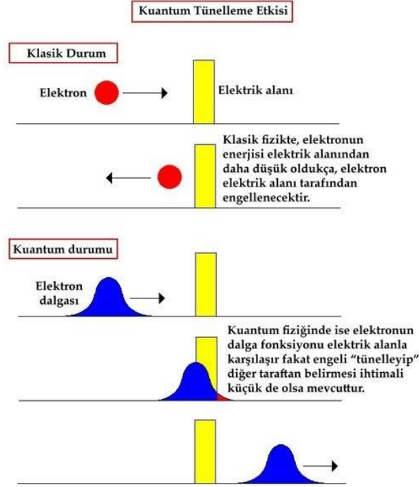
Şekil 7: Kuantum Tünellemesi (11)
