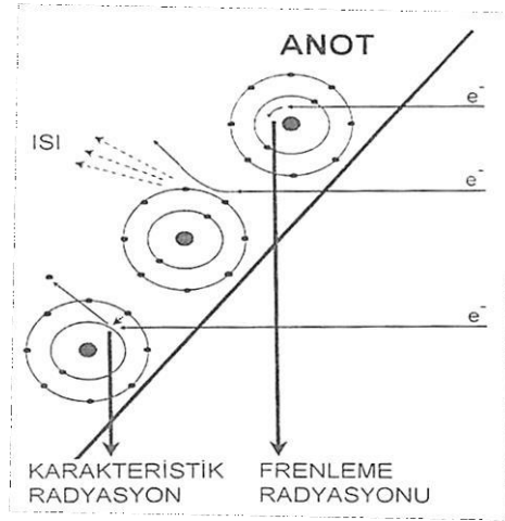
Şekil 28: X Işınlının Oluşumu (58)
