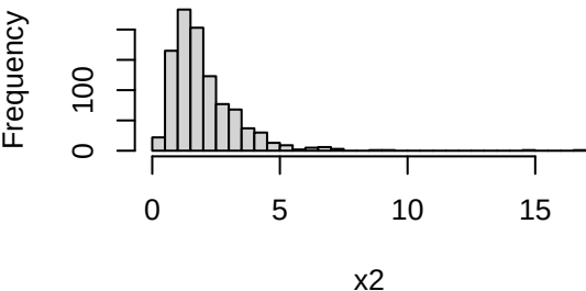
true x_2 marginal
