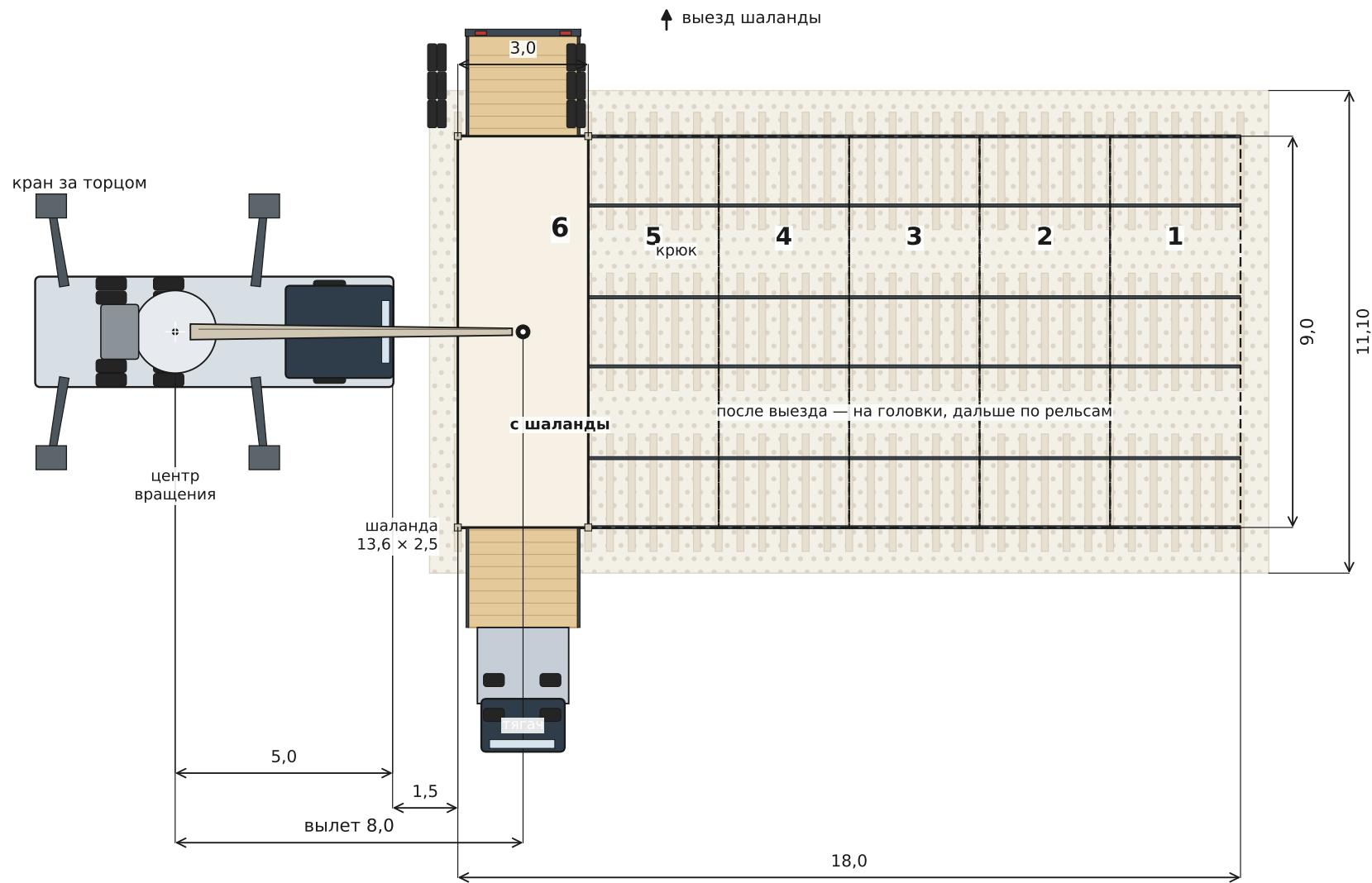
План. Шаланда перпендикулярно крану
