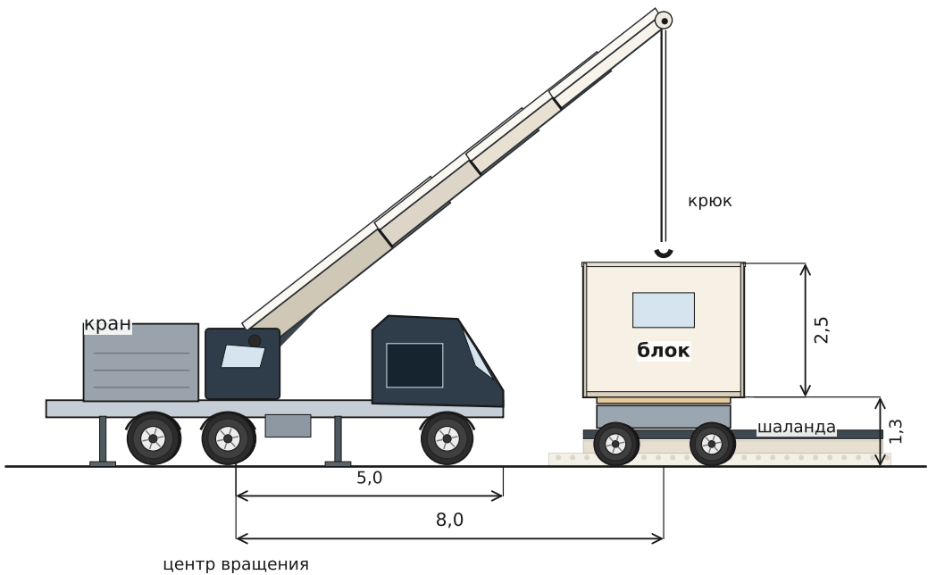
С шаланды на рельсы. Шаланда поперёк стрелы
