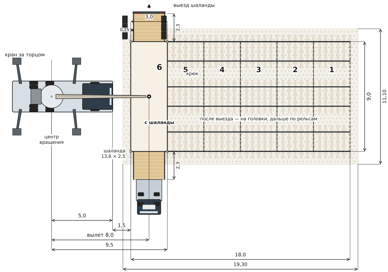
План. Шаланда перпендикулярно крану
