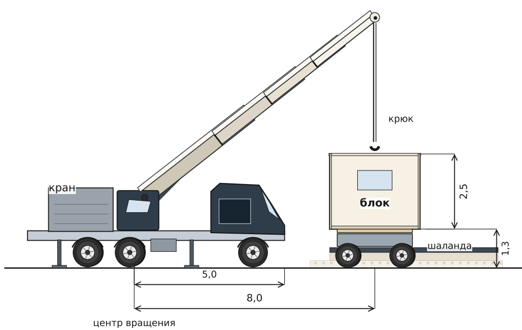
С шаланды на рельсы. Шаланда поперёк стрелы
