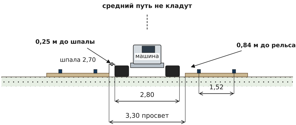
Разрез по машине. Вид с торца погрузки
