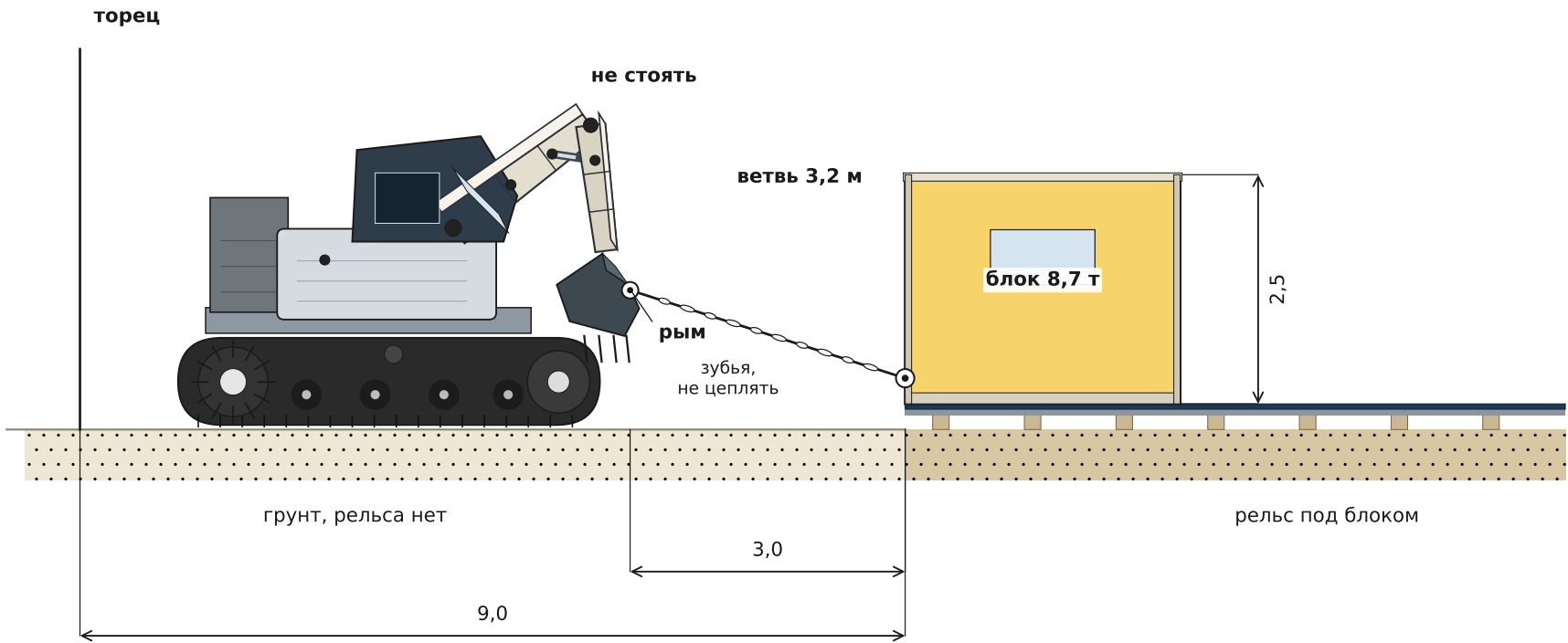
Вид сбоку. Тяга на себя, по головкам
