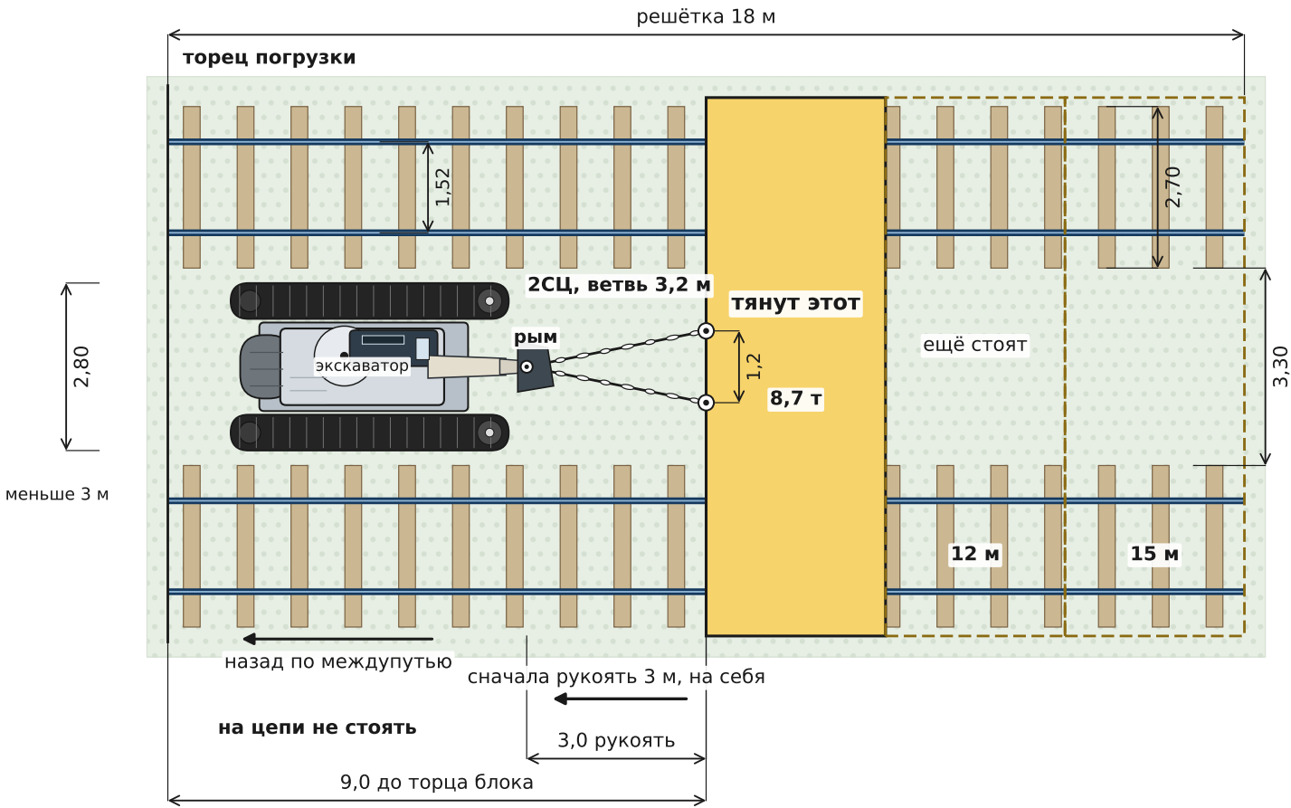
План. Два крайних пути, тяга на себя
