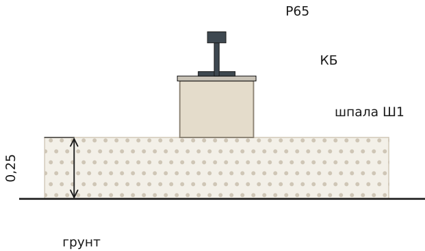
Узел рельса
