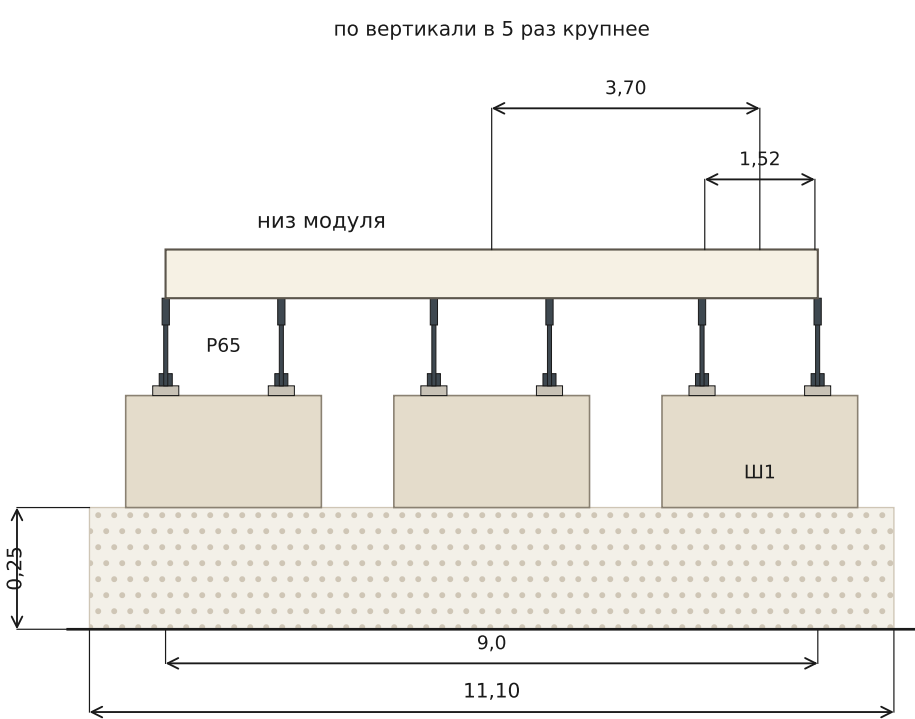
Разрез поперёк путей
