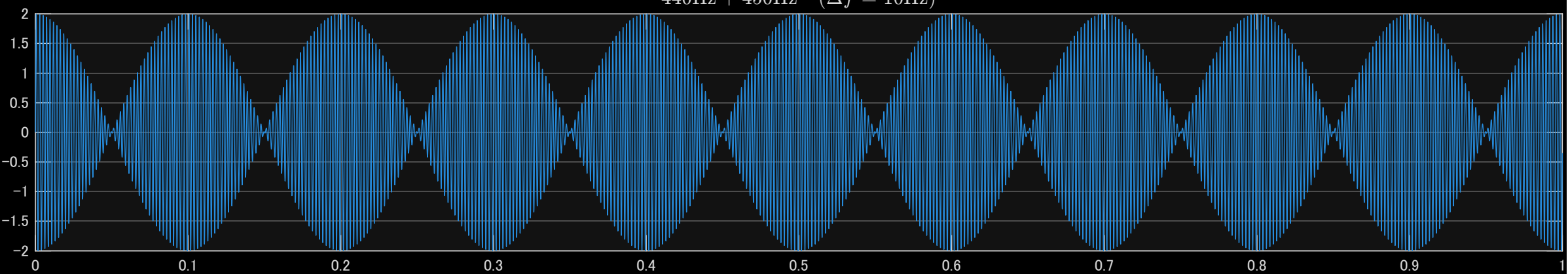
440Hz + 450Hz ( \Delta f = 10\text{Hz} )
