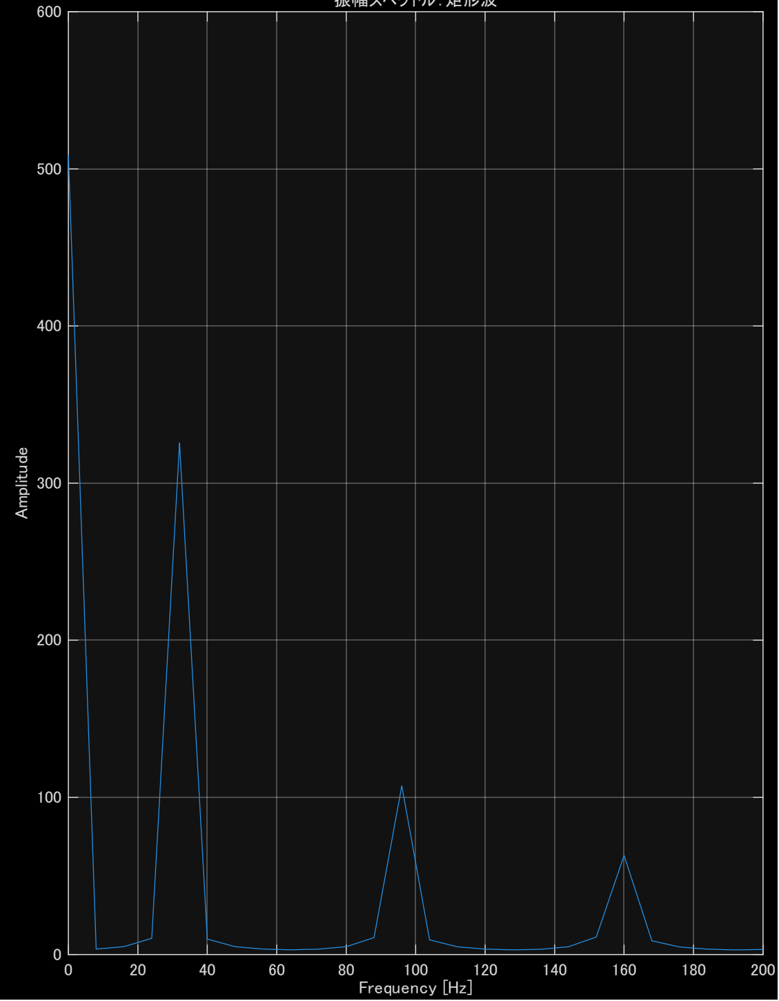
振幅スペクトル: 矩形波
