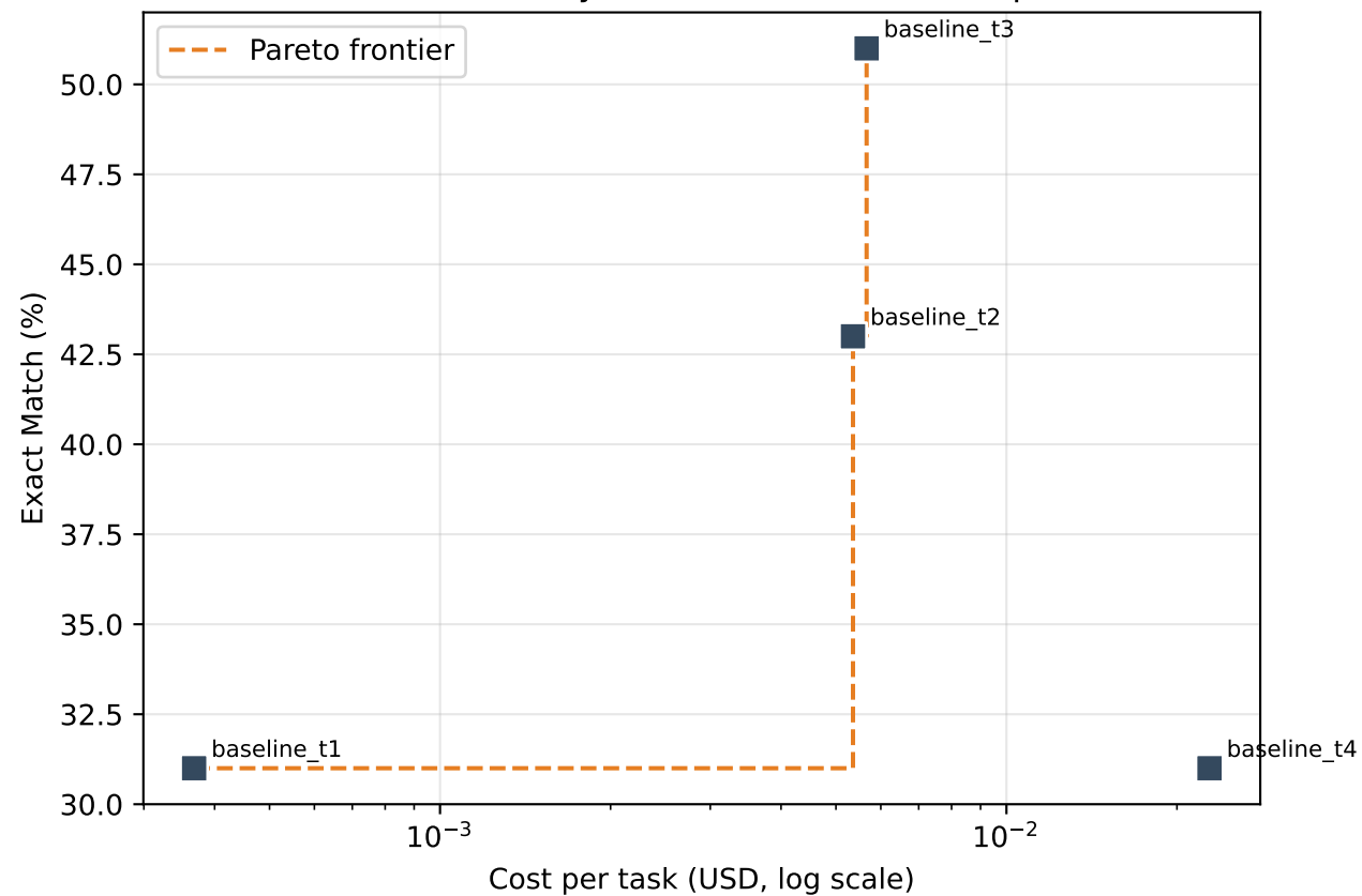
Cost vs Quality Pareto Frontier — musique
