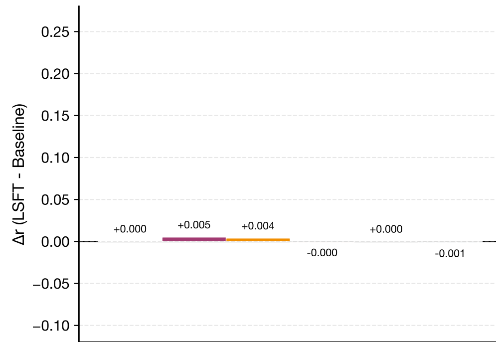
RPE1 Dataset
