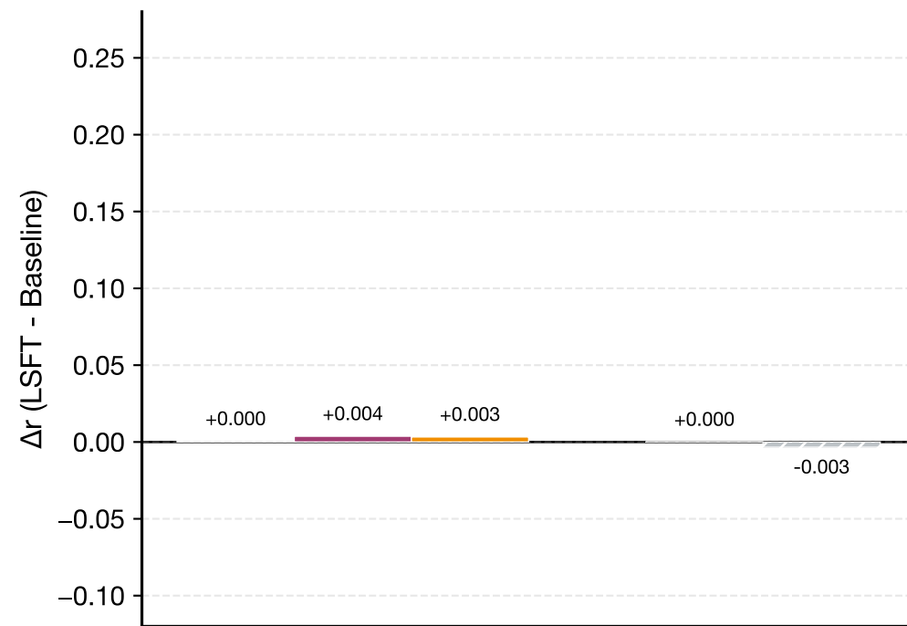
K562 Dataset
