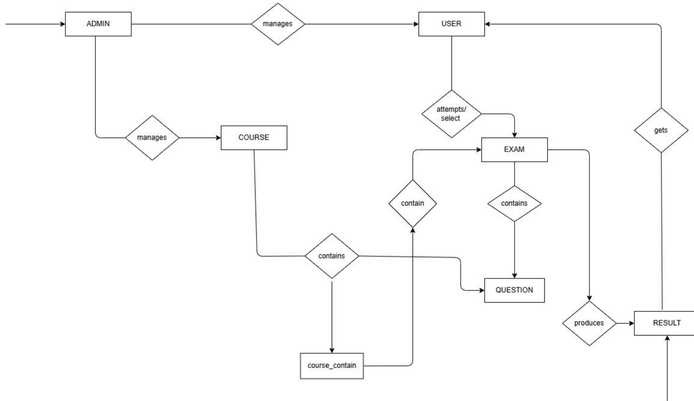
ER DIAGRAM - LEVEL 1
