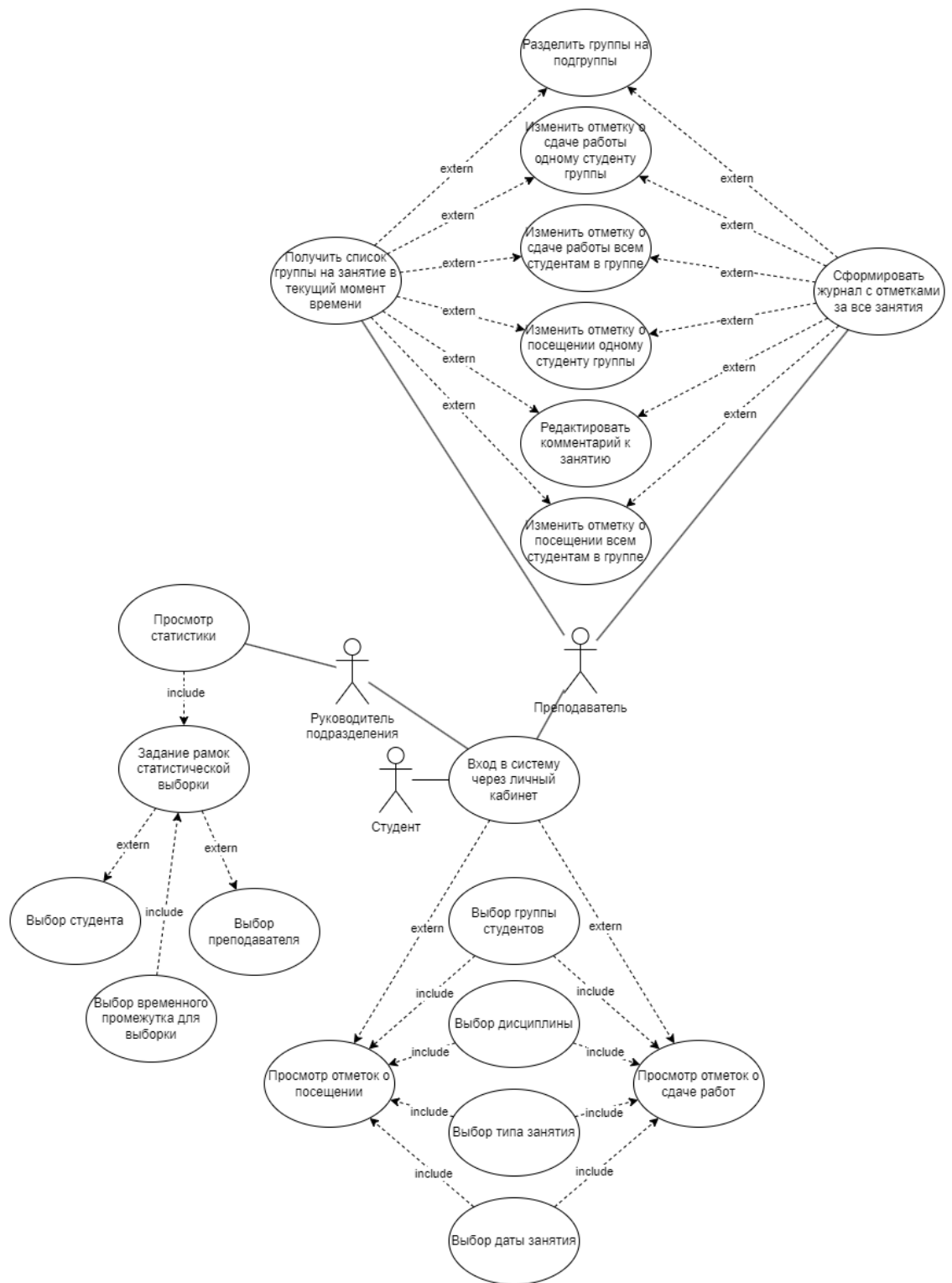
Рисунок 2.1.1 – Функциональные спецификации разрабатываемой системы
