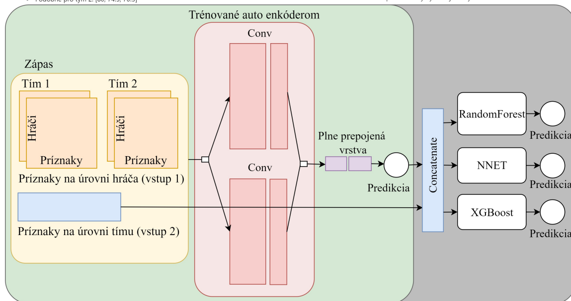
Obrázok 4.2: Schéma predikčných algoritmov systému, ktorá najprv spracováva detailné štatistiky o hráčoch. Výsledkom sú pravdepodobnosti predikovaných udalostí. Tieto pravdepodobnosti sú potom spájané s datasetom na úrovni tímov, čím vzniká komplexný vstupný dataset. Následne sa tento dataset využíva ako vstup do jedného z troch dostupných modelov, ktorý produkuje konečnú predikciu udalosti.
