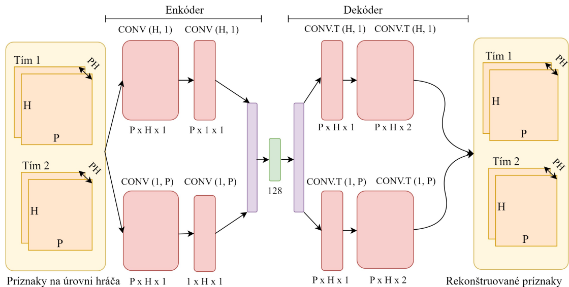
Obrázok 4.3: Konvolučná neurónová sieť tréňovaná s využitím autoenkodéra. Cieľom siete je naučiť sa efektívne komprimovať dáta do jednorozmerného vektora, pričom sa snaží zachovať maximum informácií o pôvodných zostavách hráčov jednotlivých tímov. Premenná H označuje počet hráčov v matici, zatiaľ čo premenná P reprezentuje počet príznakov pre každého hráča. Tretou dimenziou vstupných dát je premenná PH , ktorá symbolizuje posty (pozície na ihrisku) jednotlivých hráčov, pričom informácie o pozícii sú rozkopírované naprieč celým riadkom. Tento obrázok (respektíve ľavá časť) odpovedá červenej časti v obrázku 4.2
