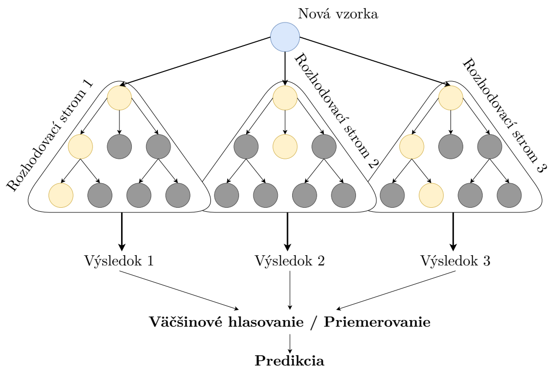
Obrázok 2.4: Schéma algoritmu Random Forest zobrazujúce kolektívne rozhodovanie viacerých rozhodovacích stromov. Každý strom dostáva novú vzorku dát a nezávisle na ostatných produkuje predikciu výsledku. Výsledné hlasovanie alebo priemerovanie týchto predikcií vedie k finálnej predikcii modelu. Tento proces znižuje variáciu a predchádza pretrénovaniu, typické pre jednotlivé rozhodovacie stromy.
