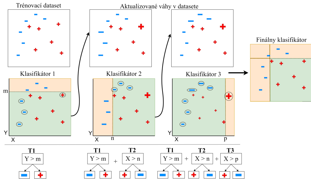
Obrázok 2.5: Sekvencia krokov ilustrujúca tréning XGBoost klasifikátora. Proces začína s trénovacím datasetom, kde každý z troch postupných klasifikátorov sa učí na vstupných dátach, pričom každý nasledujúci klasifikátor sa zameriava na nápravu chýb predchádzajúcich. Oblasť, kde každý klasifikátor zasahuje, je zobrazovaná s hraničnými čiarami ukazujúcimi prahové hodnoty ( m , n , p ), ktoré rozdeľujú priestor na regióny rozhodnutia. Finálny klasifikátor potom kombinuje výstupy všetkých predchádzajúcich stromov do jedného rozhodnutia, čo ilustruje model v poslednom paneli, kde sú rôzne regióny farebne odlíšené podľa výslednej klasifikácie.
