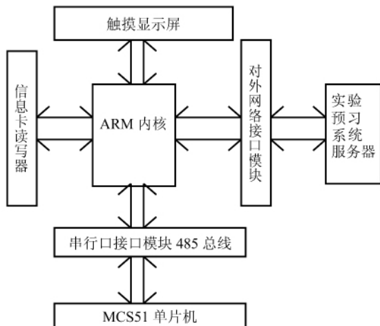
图2 硬件框图
