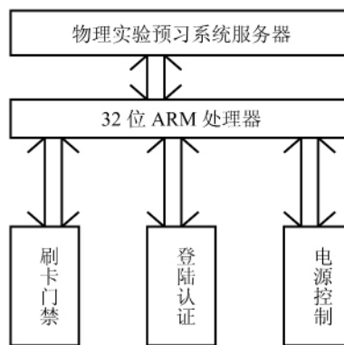
图3 预习系统服务器框图
