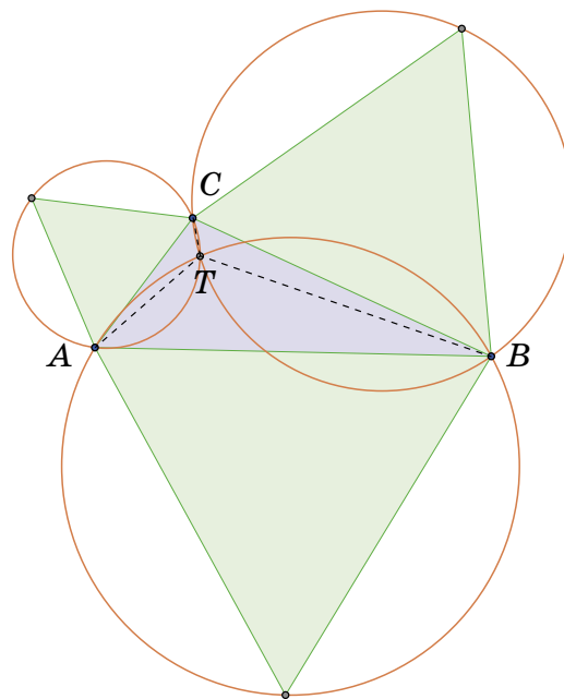
Точка Ферма – Торричелли
