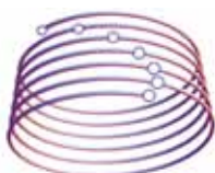
Левое дерево
