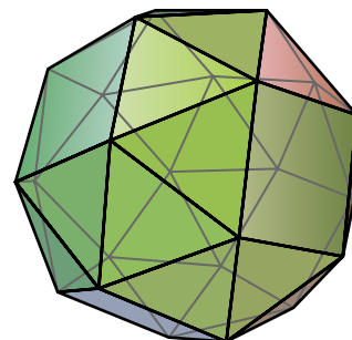
Курносый куб
