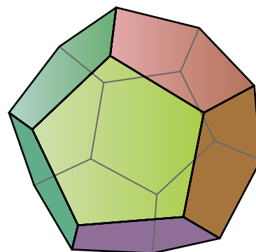
Додекаэдр
