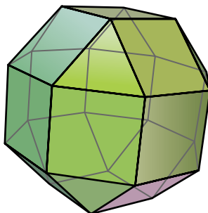
Ромбокубооктаэдр
