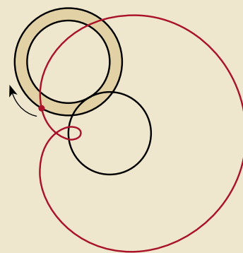
Улитка Паскаля – траектория точки обода, закреплённого на круге, который катится по кругу того же радиуса
