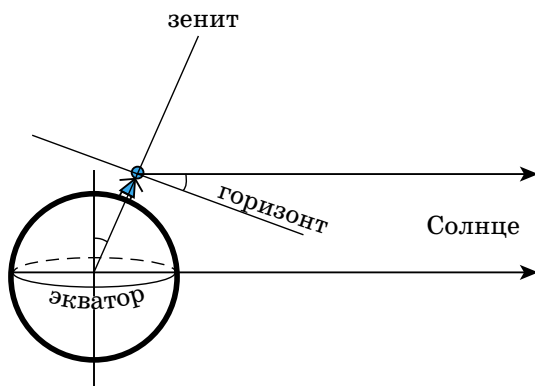
Рис. 3. Размер любой планеты во много раз меньше, чем расстояние от неё до Солнца. Поэтому можно считать, что направления на Солнце из любой точки планеты параллельны, как на этом рисунке. Высота Солнца в полдень равна угловому расстоянию от наблюдателя до полюса, то есть 90^\circ минус широта наблюдателя: углы, обозначенные на рисунке дугами, равны.
