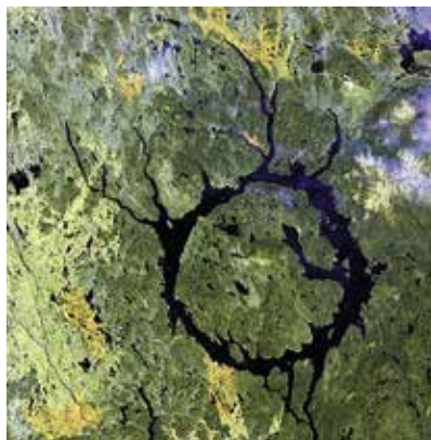
Кратер Маникуаган в Канаде, диаметр 100 км, возраст 200 млн лет
