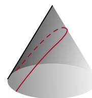
Рис. 11. Геодезические на конусе
