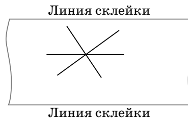
Рис. 7. Развёртка цилиндра и кусочки нескольких геодезических, проходящих через одну точку. Образующие цилиндра – горизонтальные прямые.
