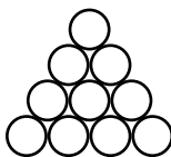
а) 4-е треугольное число 1 + 2 + 3 + 4 = 10
