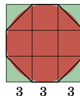
Интерпретации Фогеля (слева) и Гиймо (справа) чертежа Ахмеса
