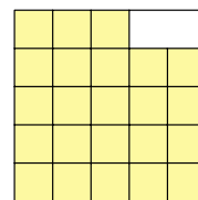
Рис. 1. Тривиальная упаковка
