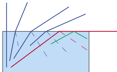
Рис. 1. Поведение выходящих лучей света на границе воды
