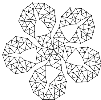
\{4, 10\} , 260 вершин
