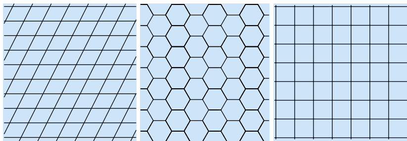
Рис. 18. Двумерные кристаллы
