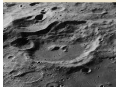
Кратер Вуда
