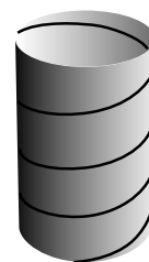
Рис. 10. Геодезическая на цилиндре
