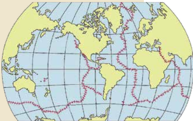
Срединно-океанические хребты показаны красным
