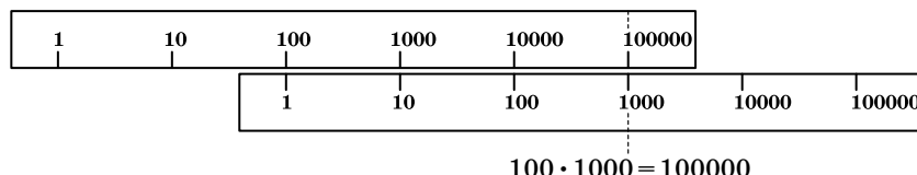
Рис. 2. Умножение степеней 10
